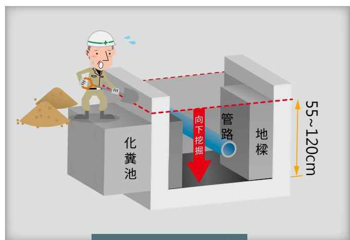
一般電梯的機坑
