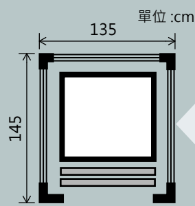
G9無機坑電梯
