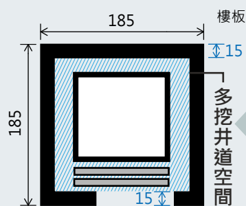
有機坑家庭電梯
